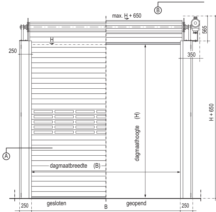
vooraanzicht
