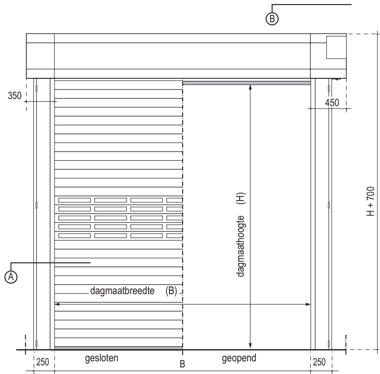
vooraanzicht
