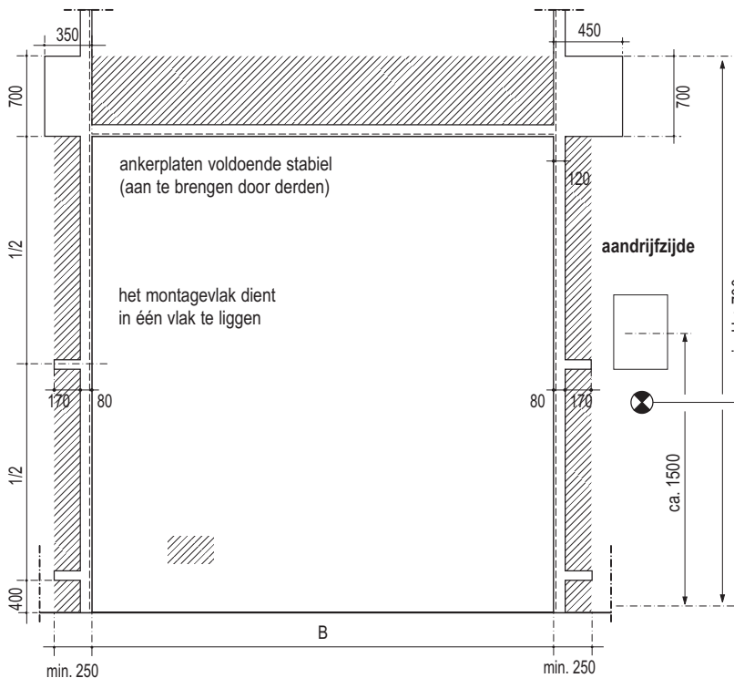
bouwkundige voorzieningen
