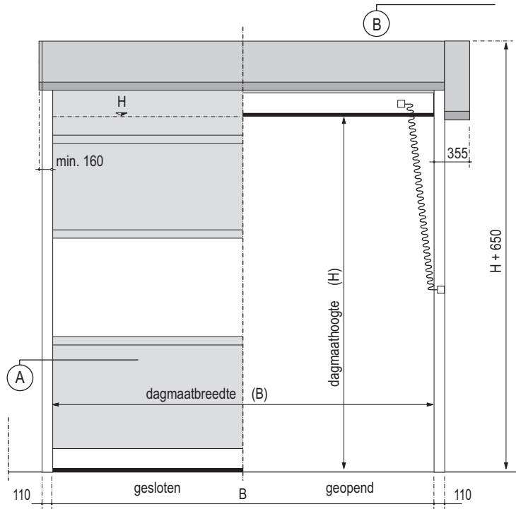
vooraanzicht
