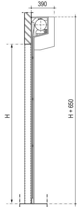
dwarsdoorsnede
