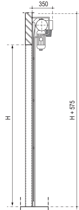
dwarsdoorsnede
