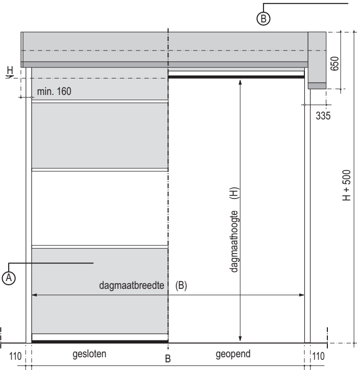
vooraanzicht
