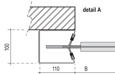
dwarsdoorsnede
