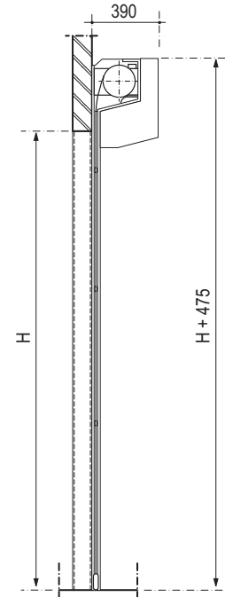
dwarsdoorsnede
