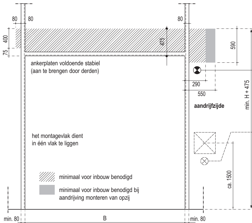
doorsnede A
