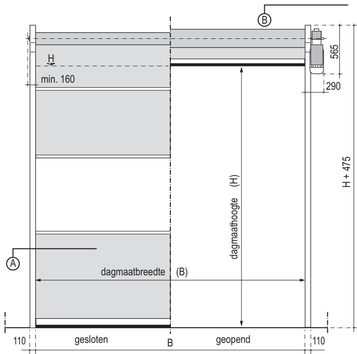
vooraanzicht
