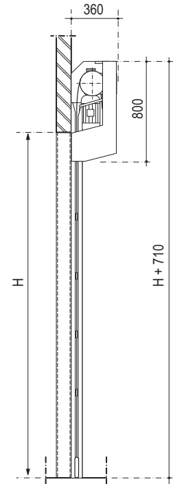
dwarsdoorsnede
