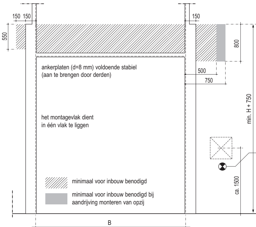
bouwkundige voorzieningen
